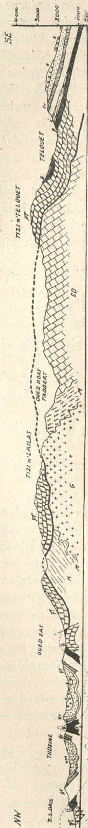
Rys. 4. Profil geologiczny przez Wysoki Atlas. Objasnienie znaków: G — granit, M — łupki metamorficzne, SD — sylur i dewon, PT — permotrias, β — bazalt, j — jura, kr — kreda, e — eocen, om — oligo - miocen. Według L. Moreta.
