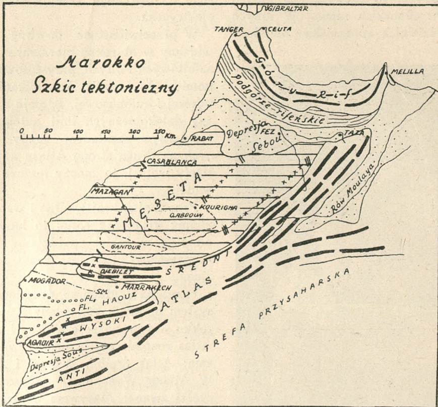
Rys. 3. Szkic tektoniczny Marokka.
