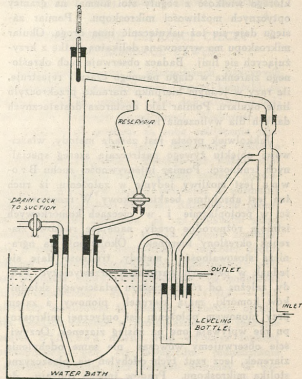
Aparat do destylacji.
