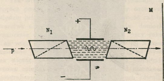
Ryc. 2. Nitrobenzol między okładkami kondensatora a pryzmatami.
