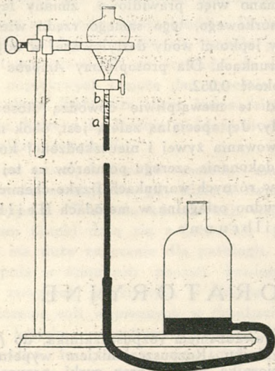
Aparat do pomiaru prędkości pary.
