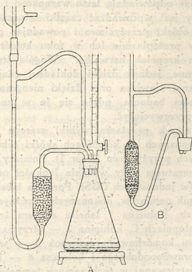
Aparat do ekstrakcji ciągłej.
