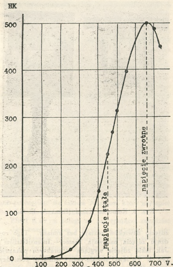
Rys. 4. Charakterystyka komórki A. E. G. Według A. E. G. Mitteilungen 1930, zeszyt 1.
