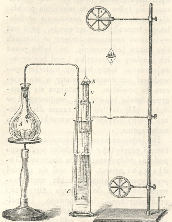
Aparat Godlewskiego do doświadczeń z oddychaniem roślin przy stałym dopływie tlenu.
