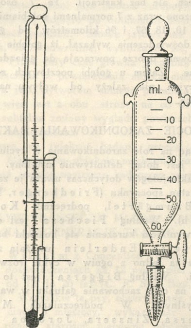
Przyrząd do oznaczania punktu topliwości.
