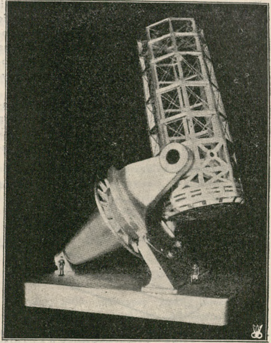
Model pięciometrowego reflektora.
