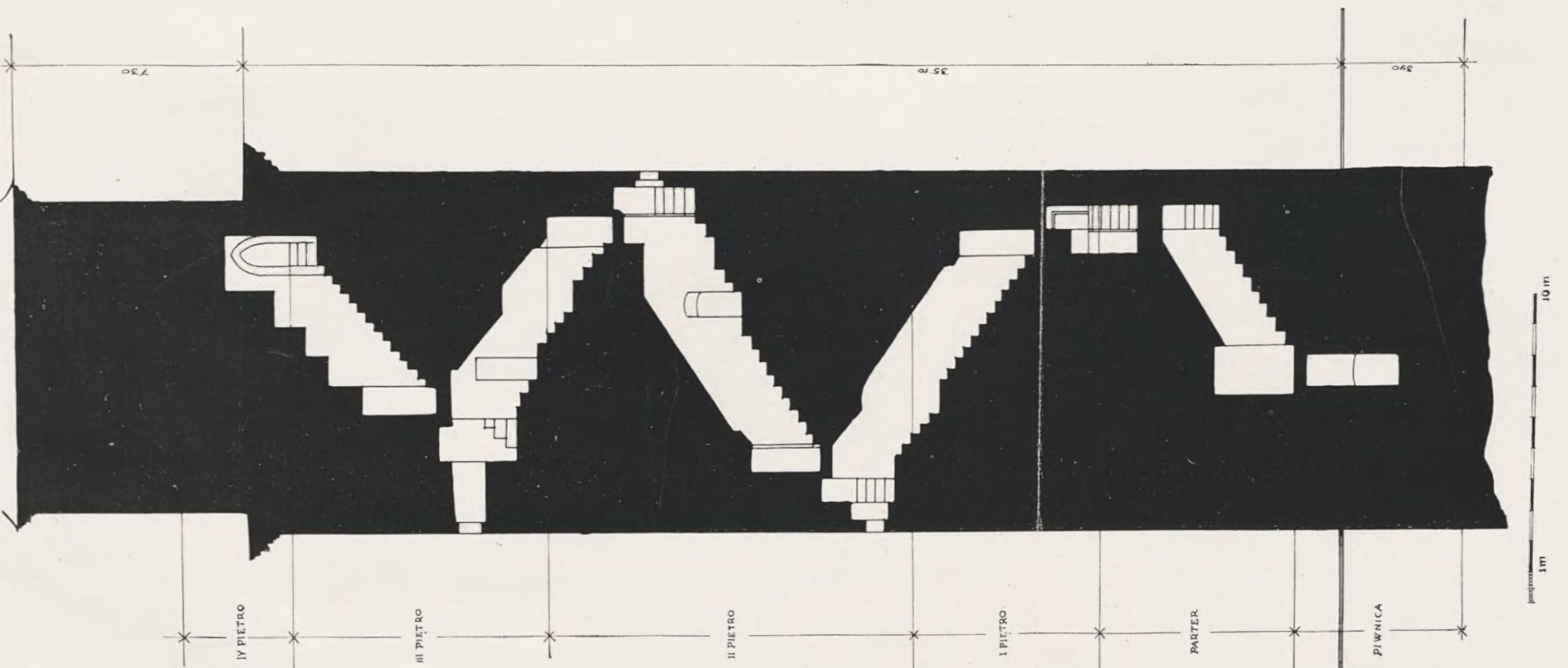
Fig. 17. Wieża ratuszowa. Przekrój pionowy po płaszczyźnie wschodnio-zachodniej.
