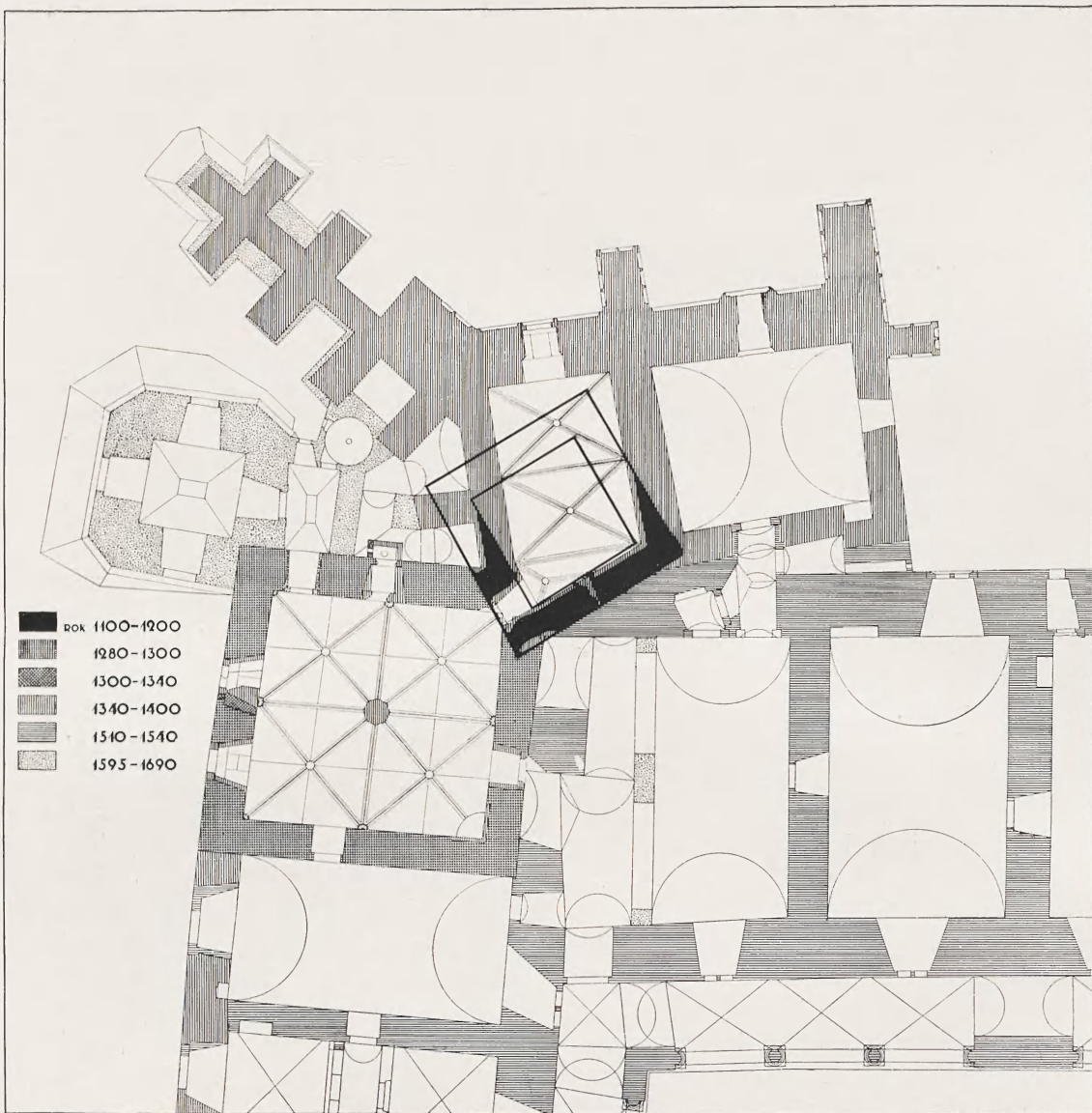
Fig. 23. Kurza Noga, plan historyczny, parter.
