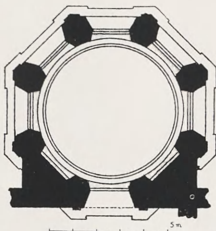
Fig. 9. Kaplica Zygmuntowska, rzut poziomy bębna (wedł. Odrzywolskiego).
