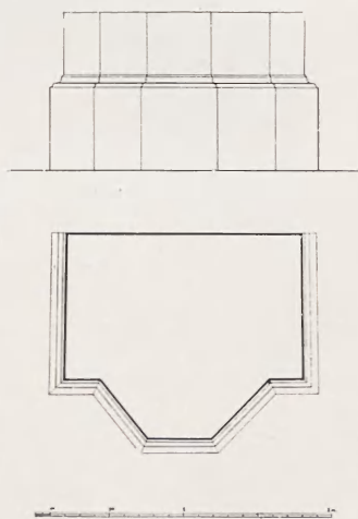
Fig. 18. Baza słupa gotyckich krużganków.
