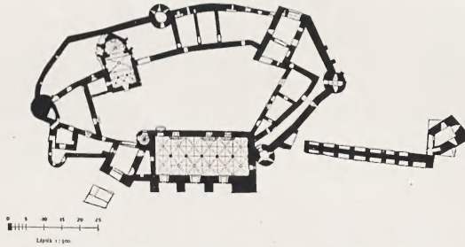
Fig. 27. Plan Zamku Vajda Hunyad. 1)
