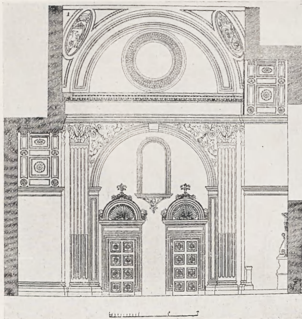
Fig. 30. Gran, kaplica kard. T. Bakocsa, przekrój (wedł. Archaeologiai Értésítő , r. 1881, zdj. S. Fellnera).
