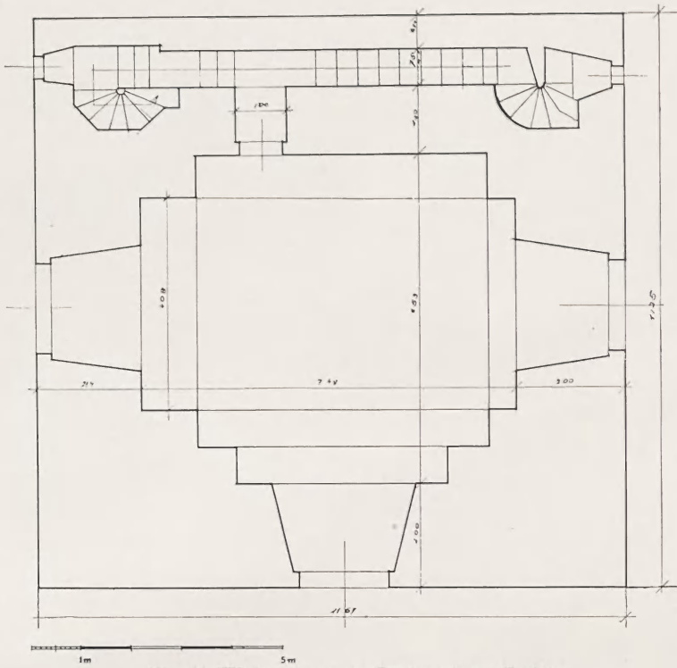
Fig. 14. Wieża ratuszowa. Rzut poziomy II piętra.
