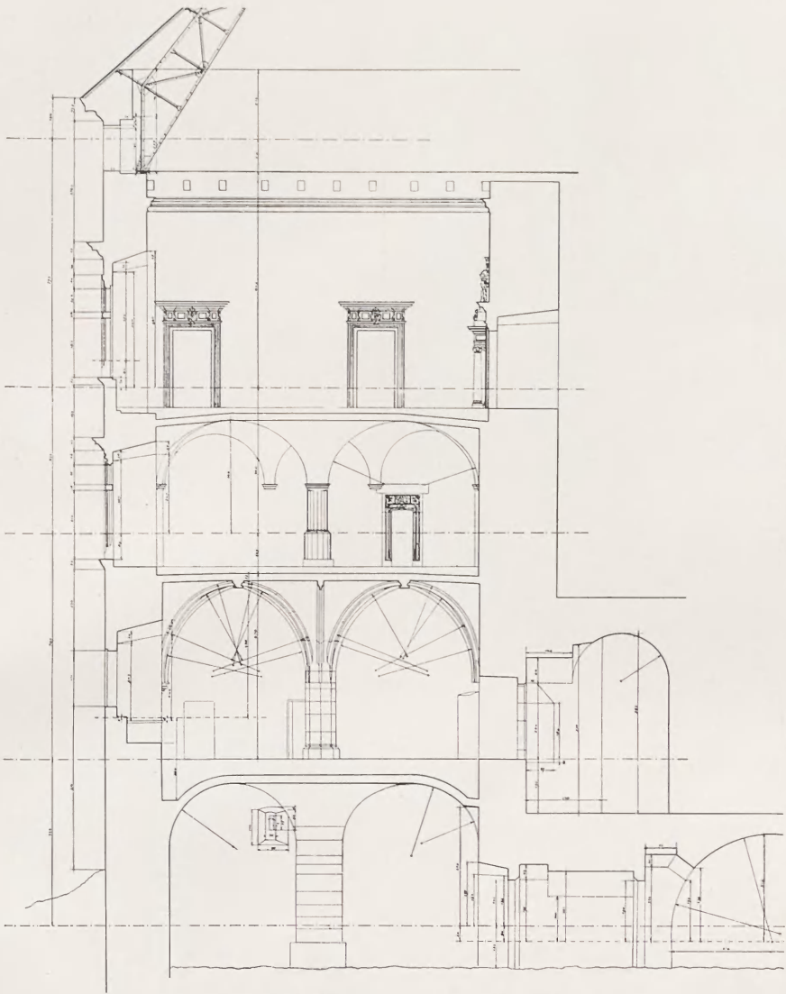
Fig. 11. Wieża Łokietkowa, przekrój stanu obecnego.
