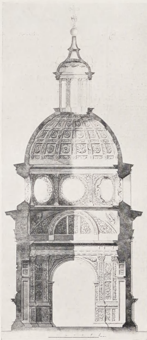
Fig. 2. Przekrój kaplicy Zygmuntofskiej. Rysunek z 2-ej poł. XVIII w. w Bibl. Uniw. Warszawskiego (fot. J. Bułhakówna).
