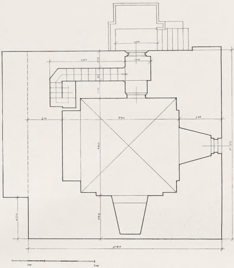
Fig. 12. Wieża ratuszowa. Rzut poziomy parteru.
