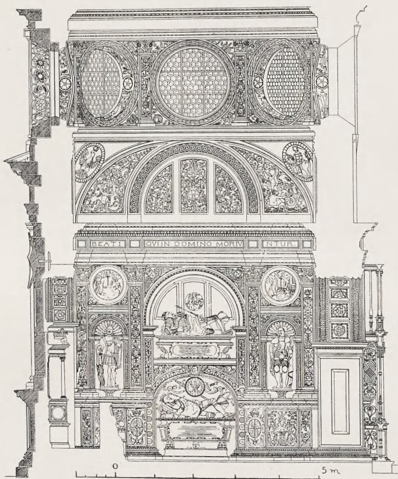
Fig. 12. Przekrój kaplicy Zygmuntowskiej do podstawy kopuły (wedł. S. Odrzywolskiego).
