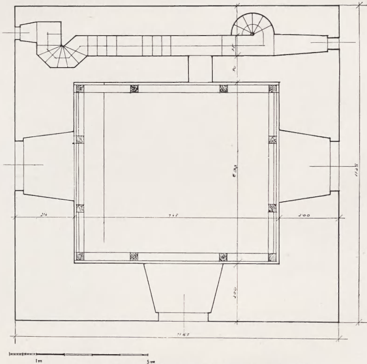
Fig. 15. Wieża ratuszowa. Rzut poziomy III piętra.
