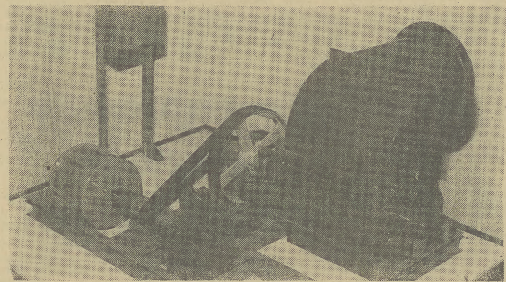
Model turbogenerators, których rodzina zaprojektowana została w krakowskim „Chemkopie”. Fot.: JAN SIUTA
