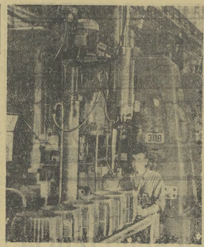
NA WĘGRZECH Fabryka maszyn i narzędzi Huty Stali i Żelaza „Csepel” wyprodukowała na zamówienie Związku Radzieckiego prototyp automatycznej linii do ciecía odlewów maszyn.
