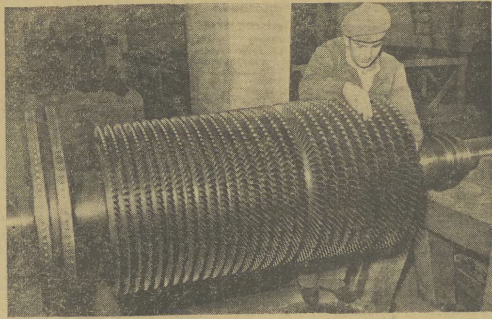
Na zdjęciu: przegląd wirnika wysokoprężnego przewoźnika montera Wilhelma Wieszczyka, CAF - fot. St. Wdowiński
