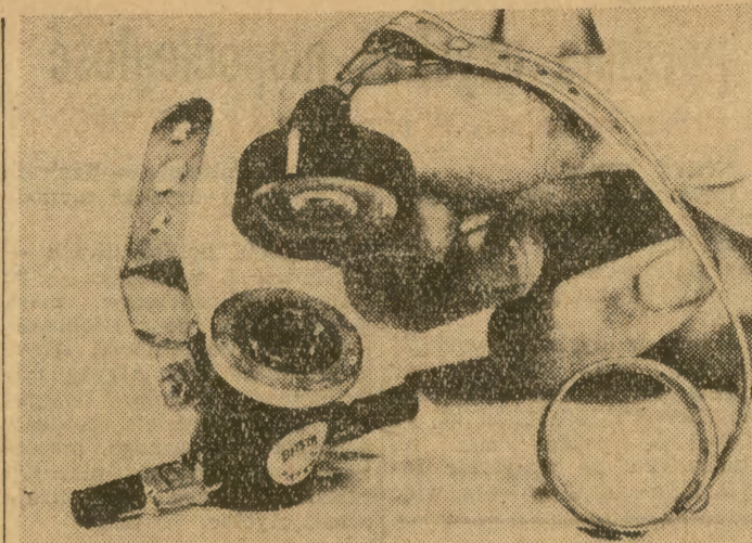
Nowy wynalazek duński — główny bezpiecznik samochodowy — zapobiega, ma w wypadku katastrofy zapaleniu się benzyny. Podłączony do głównego przewodu elektrycznego, bezpiecznik składa się z dwóch części, z których górna stanowi elektromagnes w bakelitowej osłonie. W wypadku zderzenia, nawet przy szybkości 10 km/godz., górna część bezpiecznika pęka, powodując przerwanie prądu, a co za tym idzie — uniemożliwia powstanie iskry zapaleniowej w przerwanym obwodzie, która mogłaby zapalić benzynę.
